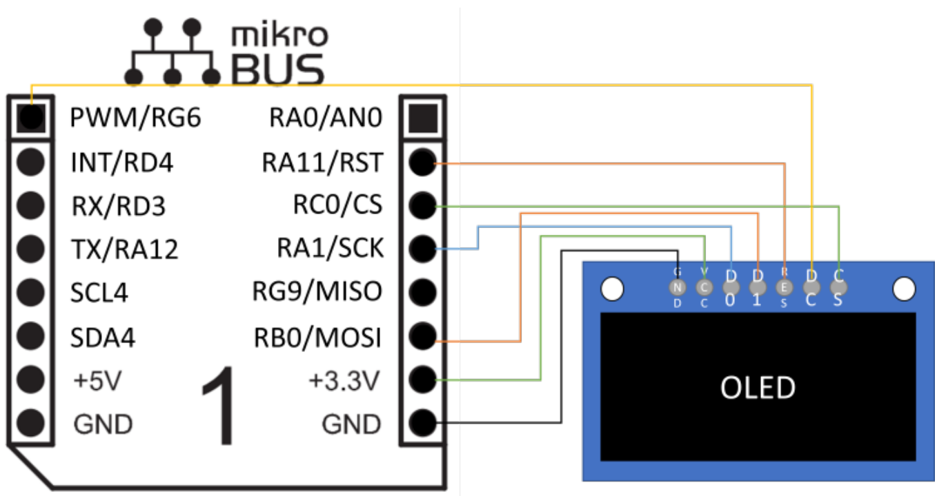
Fig. 32: Anschluss OLED
