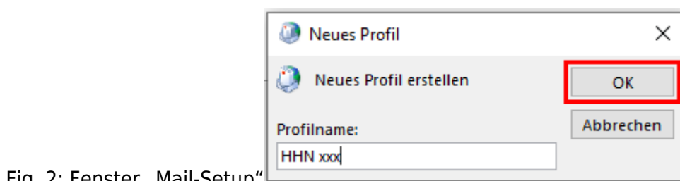
Fig. 2: Fenster „Mail-Setup“
