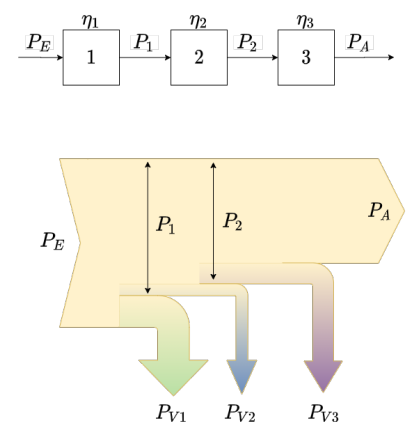
Fig. 10: Leistungsflussdiagramm
